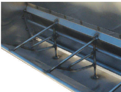
Figura 2.1: Comedero de Perfil Bajo con Divisores de Boca
